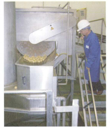
7. Lúpačka DORNOW s lúpacími valcami DORNOW R-OW- 130-A v prevádzke na spracovanie zemiakov.
