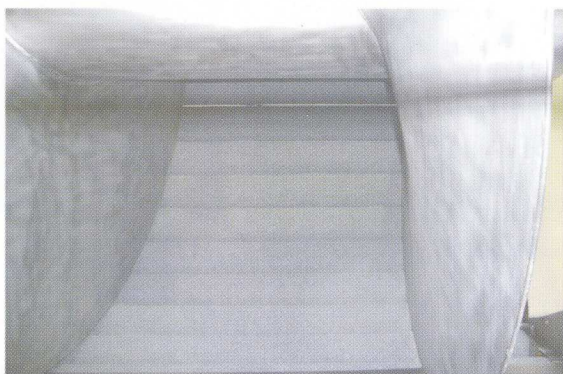
Pohľad do lúpačky s lúpacími valcami, typ R-OW 190-A1, ktorá je vybavená 14 karborundovými valcami o priemere 150 mm, dĺžka valcov je 4.000 mm. Priemer dopravného šneku je 1.900 mm.
